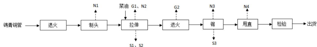
图 3.5-1 项目生产工艺流程图
